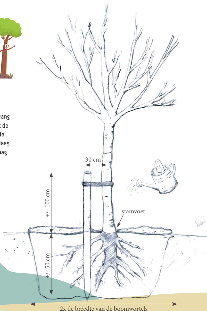
ILLUSTRATIE EN AFMETINGEN MBT DE AANPLANT VAN EEN HOOGSTAMBOOM
